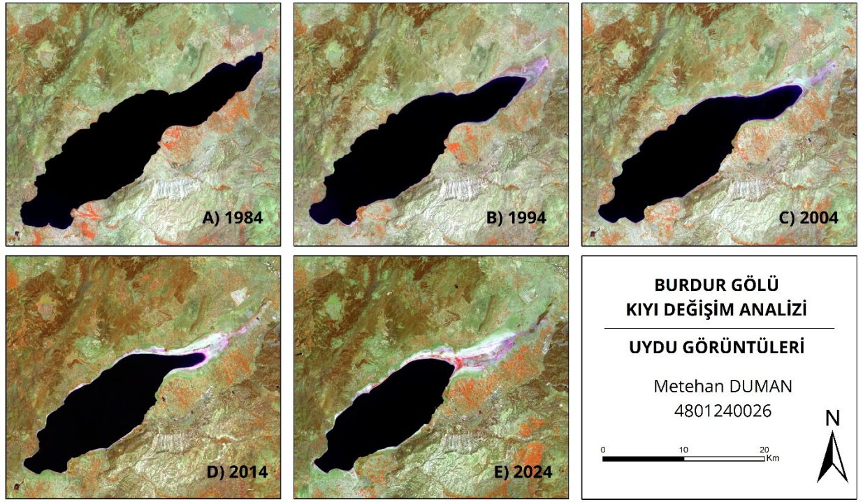
Şekil 2: 10 Yıllık Periyotlarla Burdur Gölü
